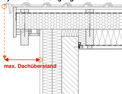
Systemskizze Ortgang
