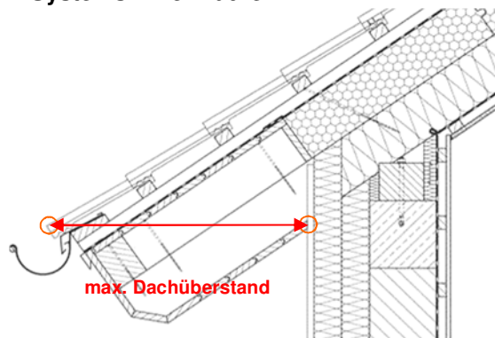
Systemskizze Traufe
